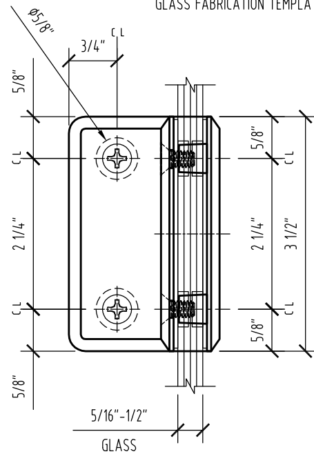
GLASS FABRICATION TEMPLATE DOOR
