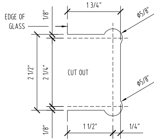
GLASS FABRICATION TEMPLATE DOOR
