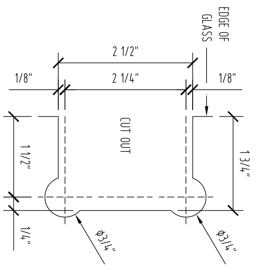
DOOR GLASS FABRICATION TEMPLATE
