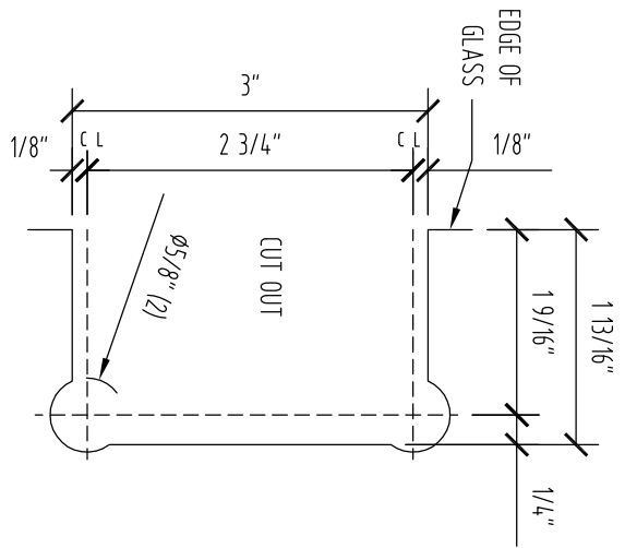
DOOR TEMPLATE
